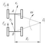
Рисунок 1 – Бортовой способ поворота колёсного трактора
